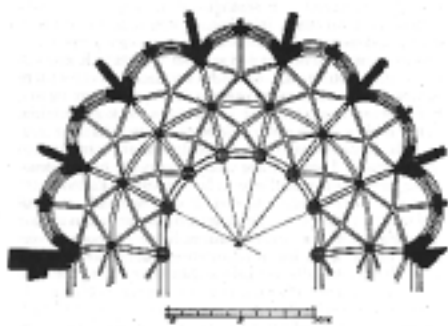
Choro abbatiale di St. Denis. Pianta del coro.
