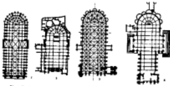
41. Piani di crociere gotiche: 1, Parigi; 2, Toledo; 3, Bourges; 4, Clermont.
