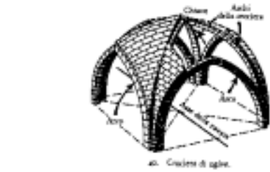
40. Crociera di ogiva.
